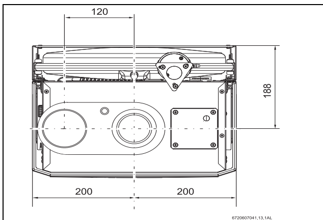
Fig. 2 Vista dall'alto con sdoppiatore 80/80 mm (acc. AZ 430)
